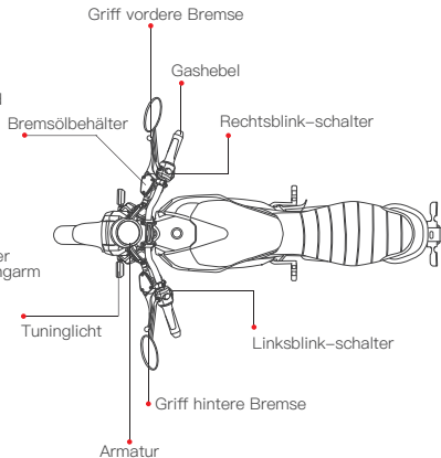
Draufsicht
